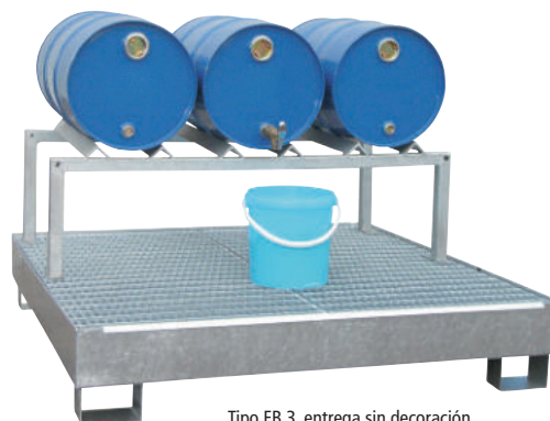
Tipo FB 3, entrega sin decoración
