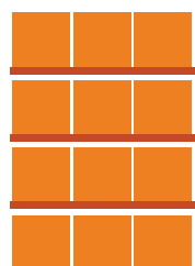
Sección adicional 1 sección por cada 1800 mm 12 espacios para palets
