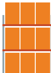
Sección base 1 sección por cada 2700 mm 9 espacios para palets
